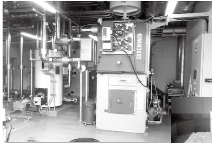
木質チップボイラー
