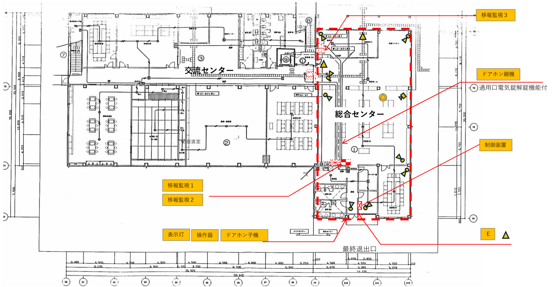
平面図1階
