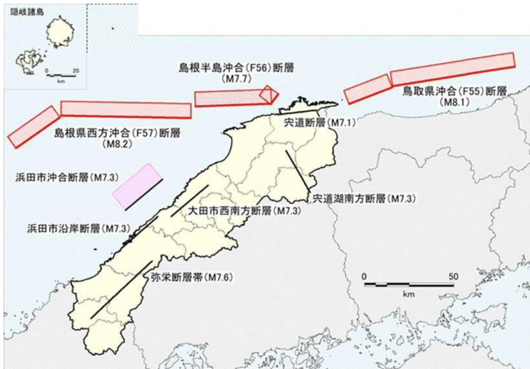
出典：出典：島根県地域防災計画（島根県 令和2年3月） 図 1-9 地震動の想定を対象とした地震の断層位置
