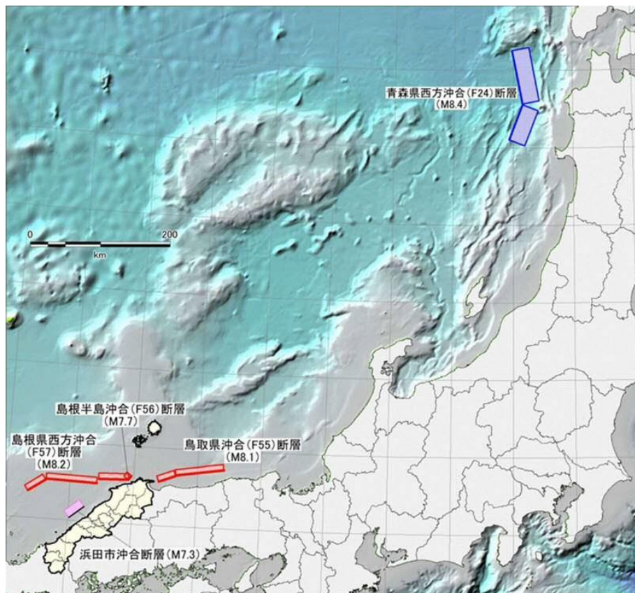
出典：出典：島根県地域防災計画（島根県 令和2年3月） 図 1-10 津波の想定を対象とした地震の断層位置
