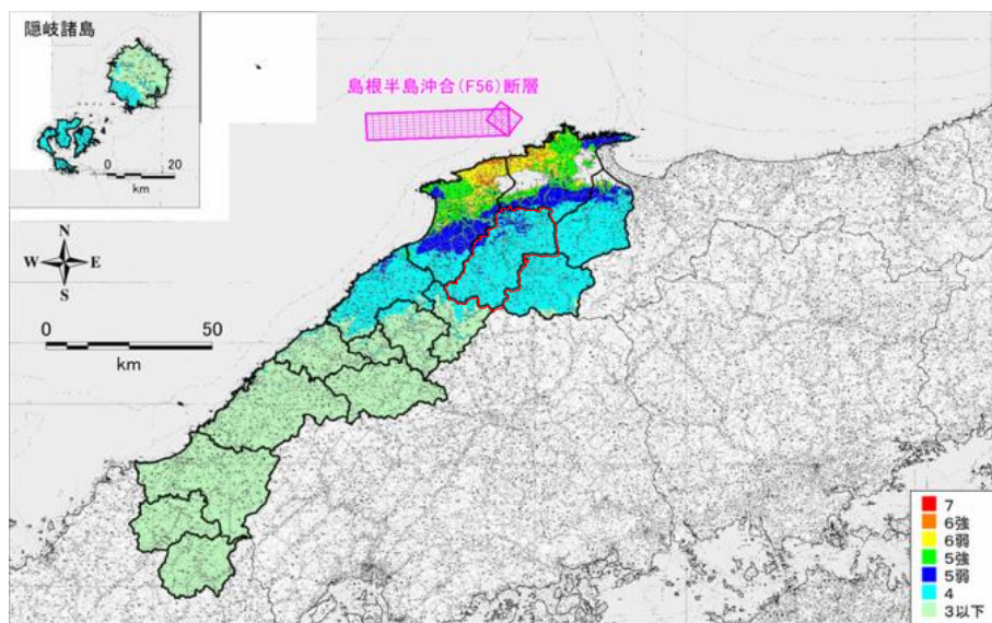
図 1-14 島根半島沖合（F56）断層の地震における地震動分布
